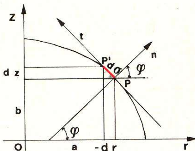
Fig. 2 - L'ellisse meridiana.
