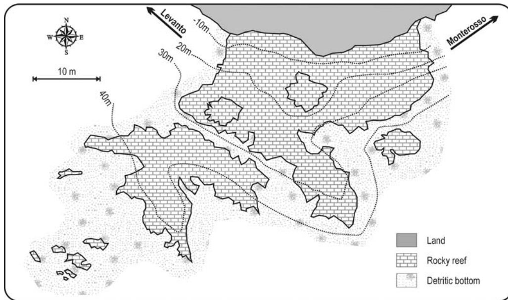
Fig. 1 - Gross morphology of the shoal off Punta Mesco (from Salvati 1997, modified). Morfologia approssimativa della secca di Punta Mesco (da Salvati 1997, modificata).
